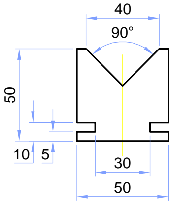
مسقط أمامي
