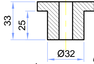
مسقط أمامي
