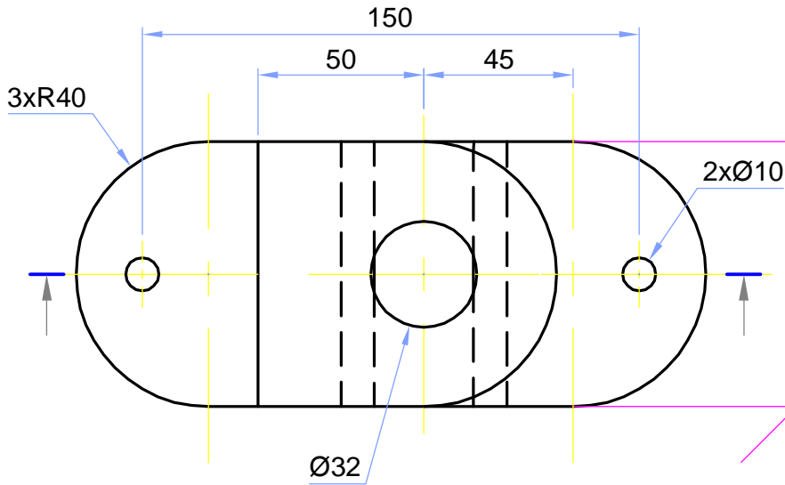
مسقط أمامي
